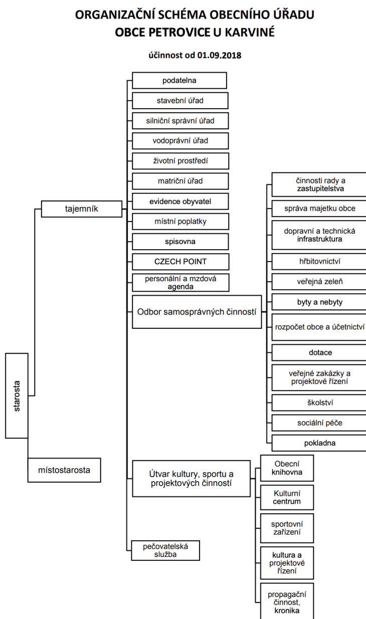
Obrázek 1-7 Organizační schéma
