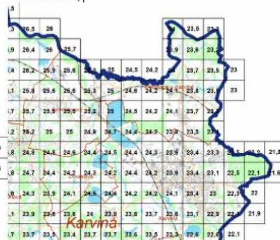
Oxid dusičitý
